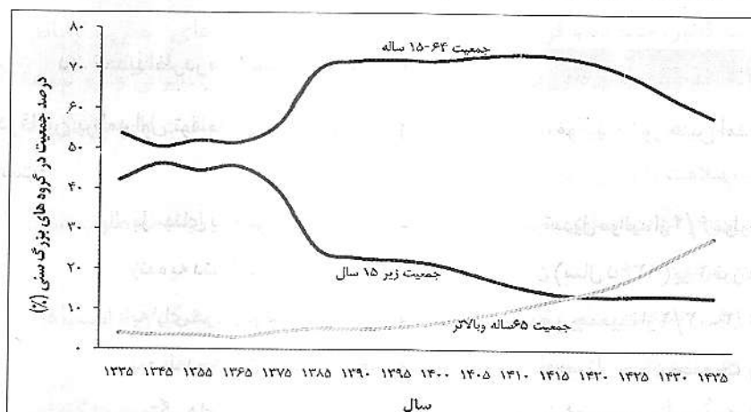
نمودار (۵): پنجره جمعیتی ایران ۱
